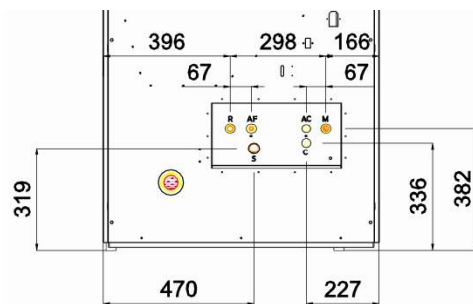
USCITA FUMI D. 100 mm Fumes outlet d. 100 mm
