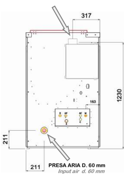
USCITA FUMI D. 100 mm Fumes outlet d. 100 mm
