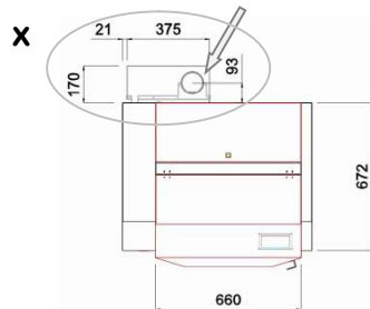
USCITA FUMI D. 100 mm Fumes outlet d. 100 mm
